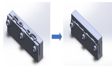
ภาพที่ 8 แบบโมเดล 3D จิ๊ก ฟิกซ์เจอร์
