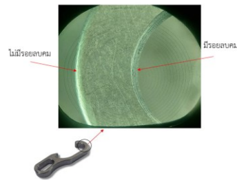
ภาพที่ 4 ตรวจสอบชิ้นงานบนกล้องไมโครสโคป (Microscopes) จุดที่ส่งผลทำให้ชิ้นงานเสีย
