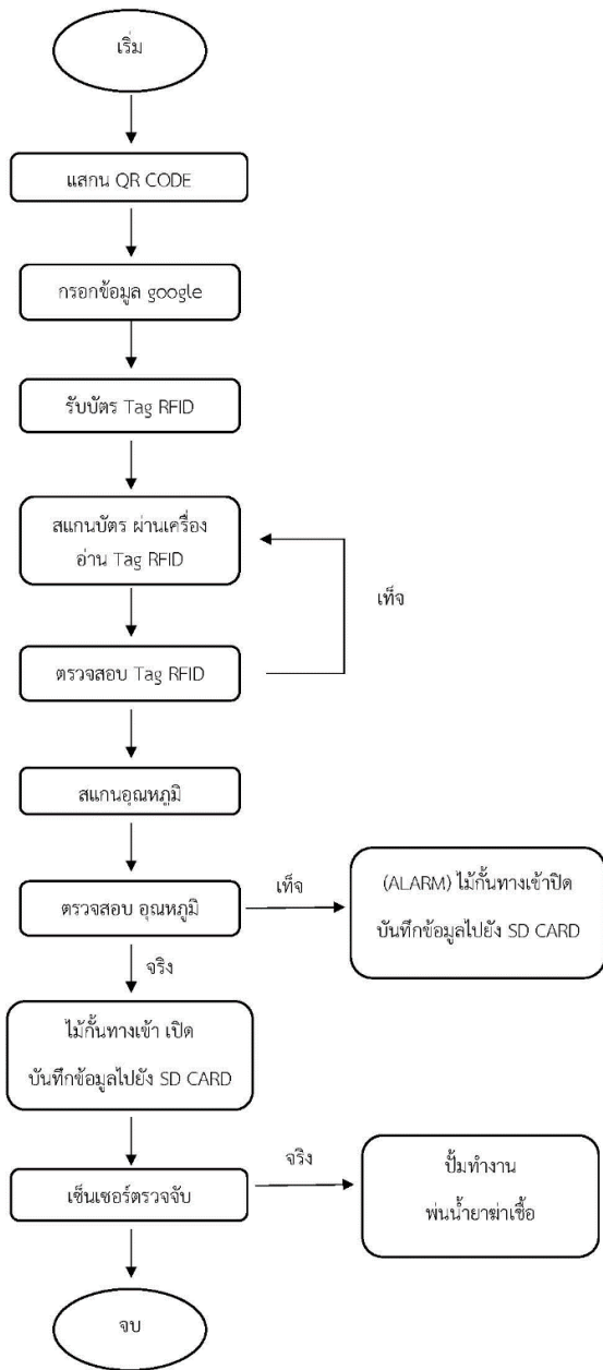
รูปที่ 4 ผังงานการทำงานของตู้ฆ่าเชื้อไวรัสโคโรนา (Covid-19)อัจฉริยะแบบไฮบริด
